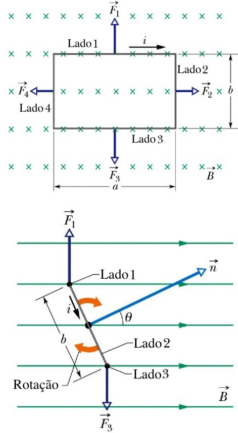
Figura 6.8: Força e torque sobre uma espira de corrente. (Halliday)
