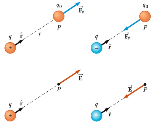
Figura 1.2: Campo elétrico. (Serway)
